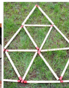
Streichholzspiele
